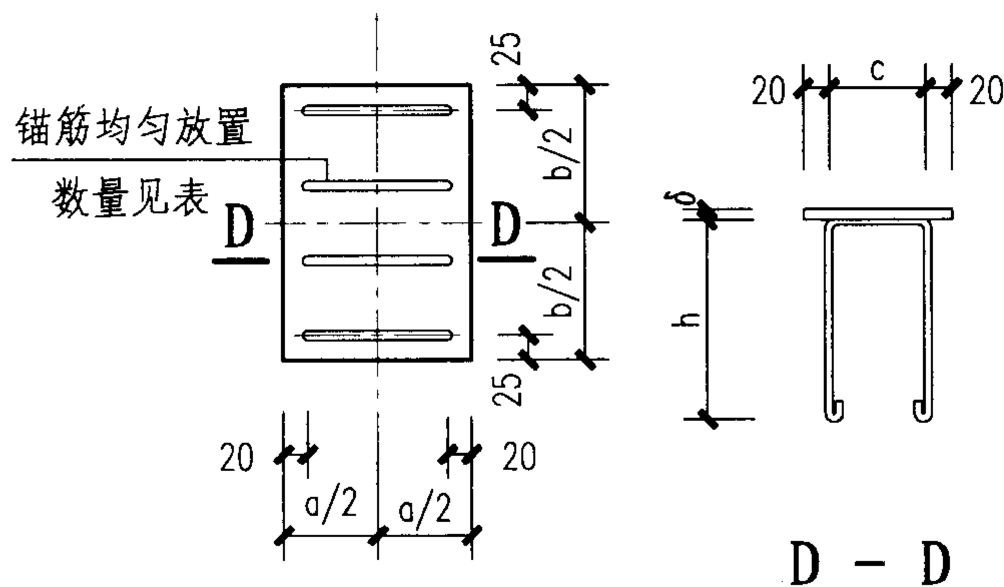
底板
