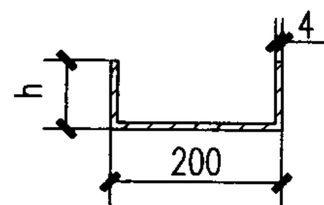
铭牌支座详图
