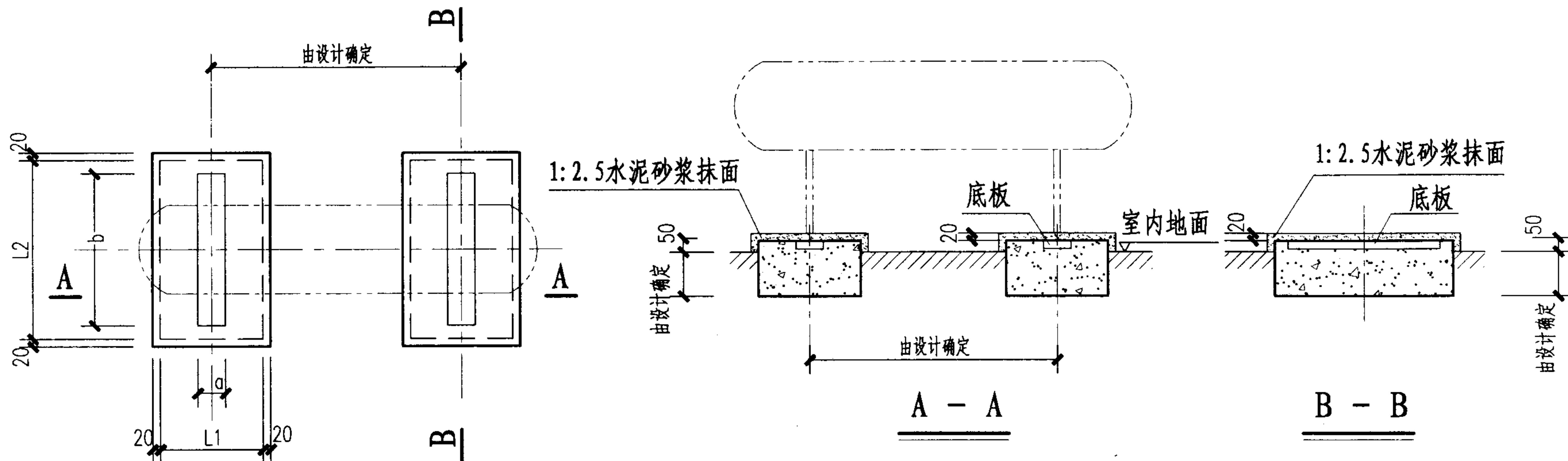
平面图
