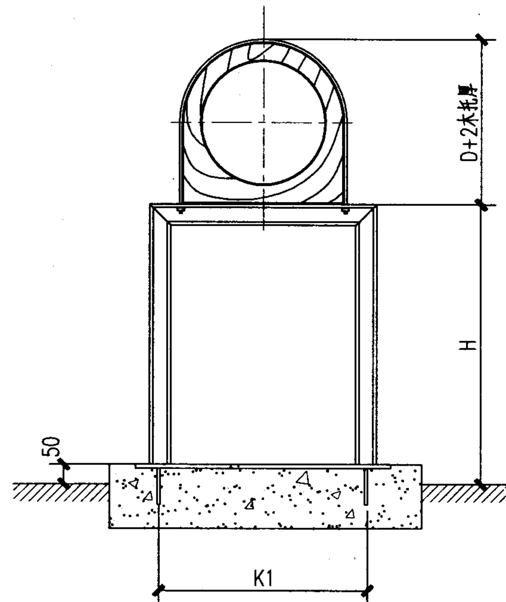
保冷支架图
