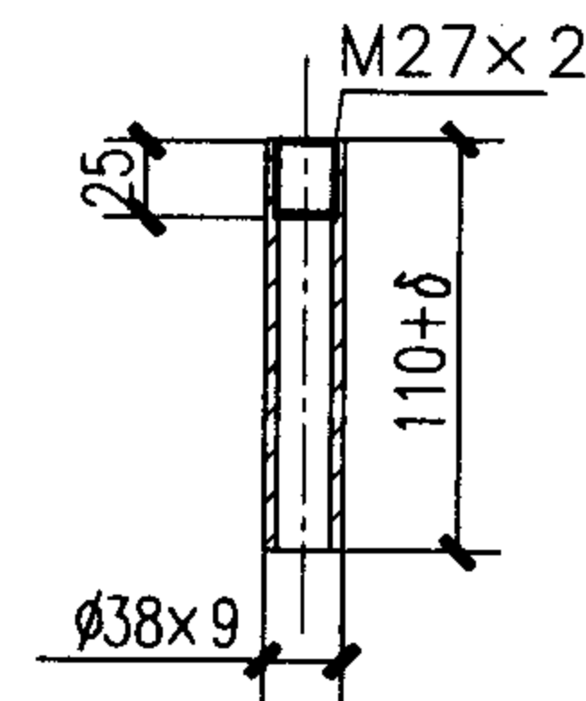
压力表接管详图
